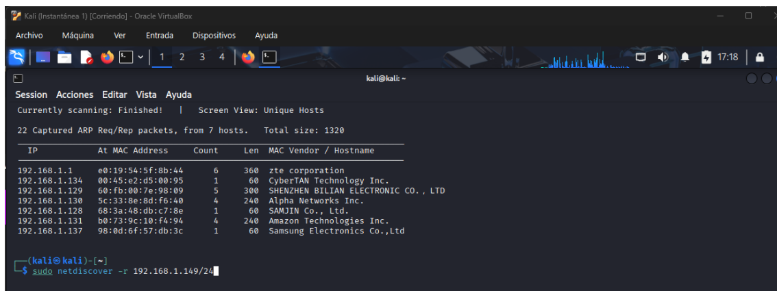
Ilustración 7 -NetDiscover
