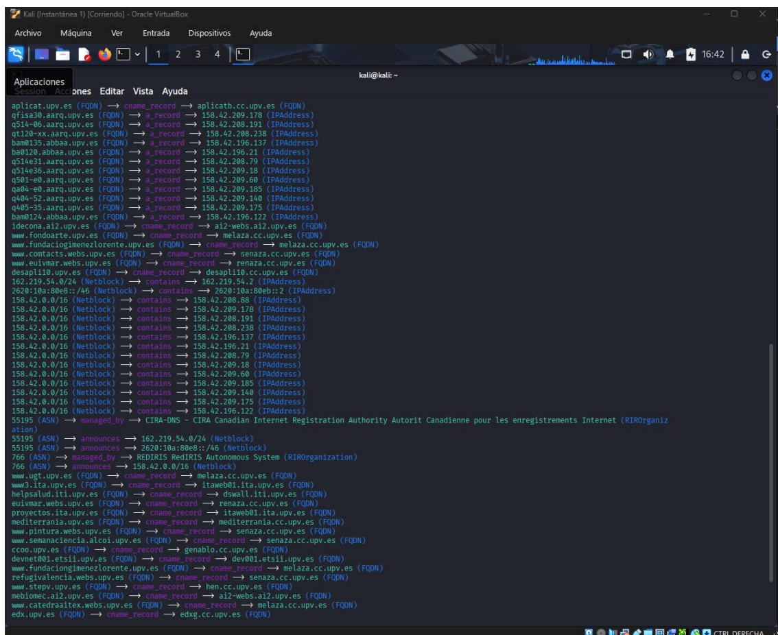
Ilustración 6 - Ejecución 'amass'
