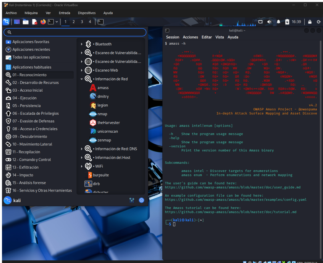
Ilustración 5 - Aplicación 'amass'
